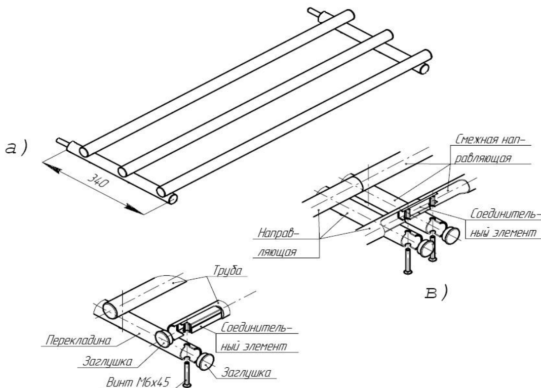
Рис. 7. Направляющая для подносов
