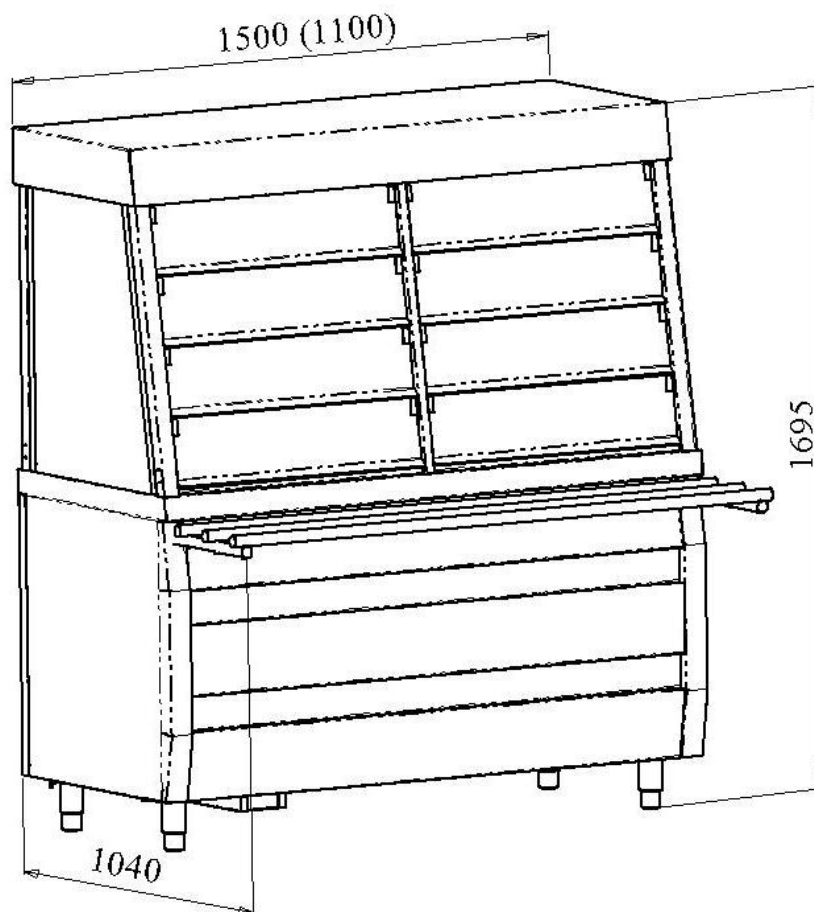
Рис.1 3ПВ-15/7Н (3ПВ-11/7Н) – комплектация с декоративной панелью и направляющей для подносов
