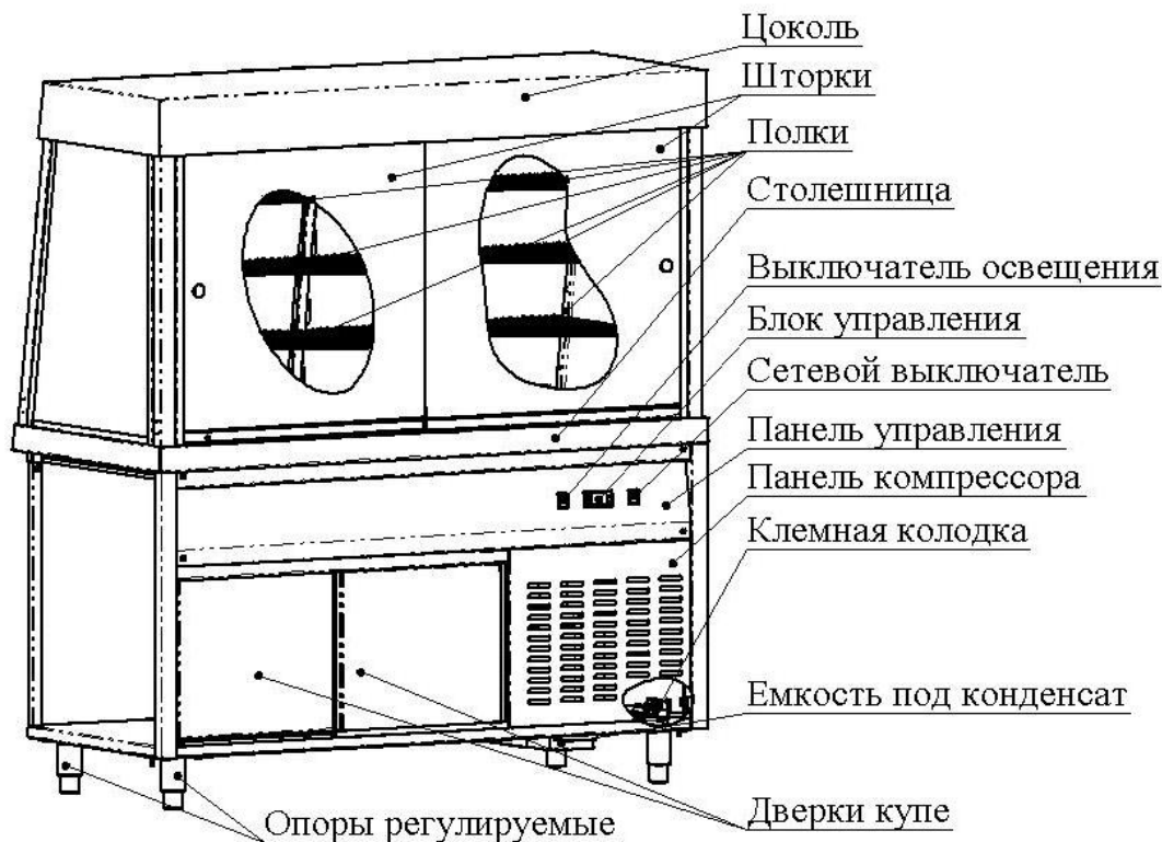
Рис.3 – Внешний вид изделия
