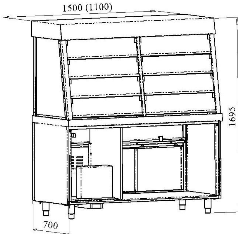
Рис.2 3PB-15/7H (3PB-11/7H) – модуль
