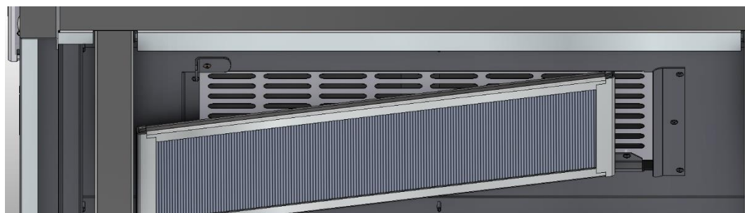
Рис. 6. Извлечение жирославливающего фильтра
